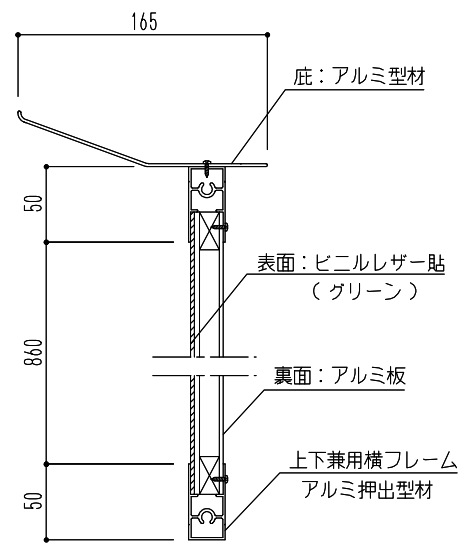
A-A 断面図
