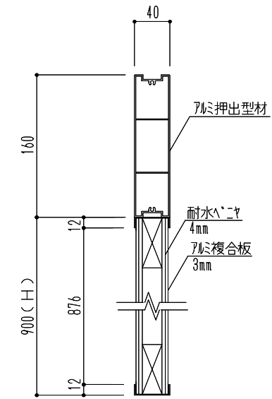
A-A部 断面図
