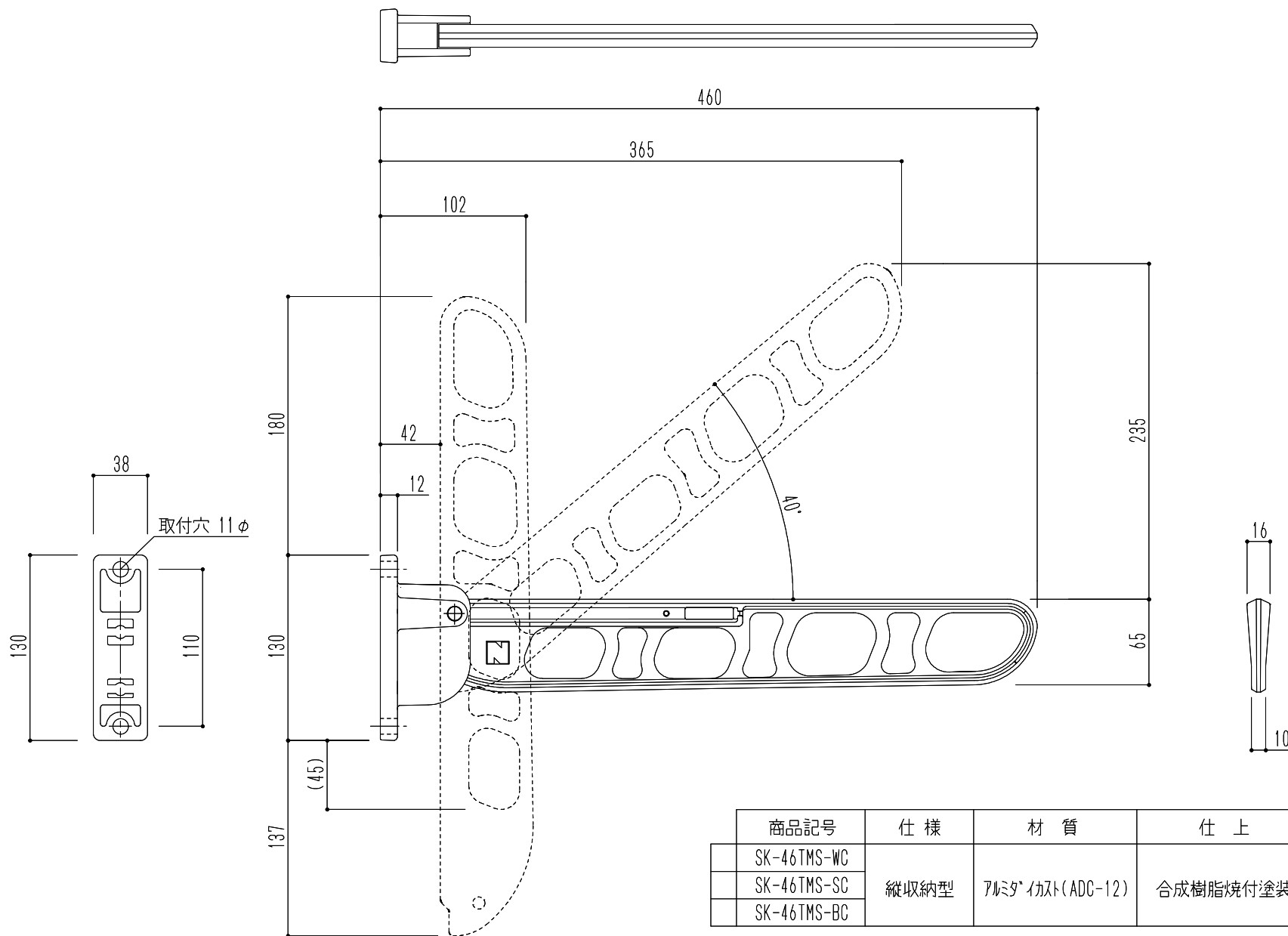
図面名 SK-46TMS-WC/-SC/-BC アルミダイカスト物干金物(縦収納型)
