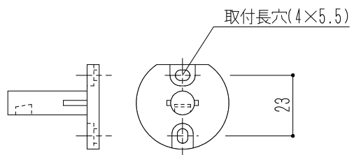
座金詳細
