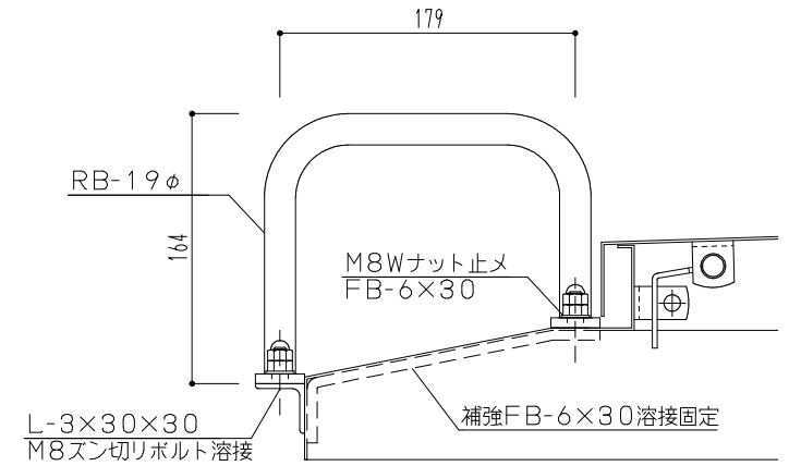
手摺取付部 詳細
