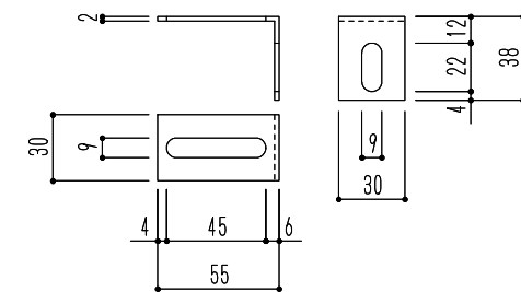
取付ブラケット詳細
