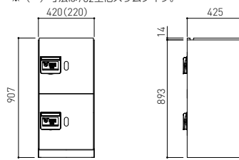
図例 SK-CBX-402型 ※ ( ) 寸法は702型他スリムタイプ。
