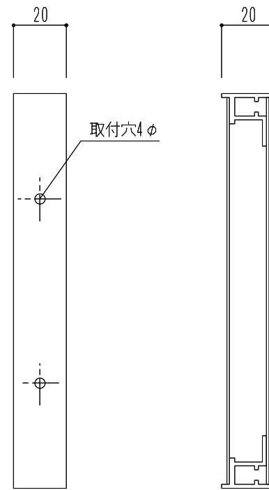
断面図
