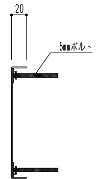
断面図
