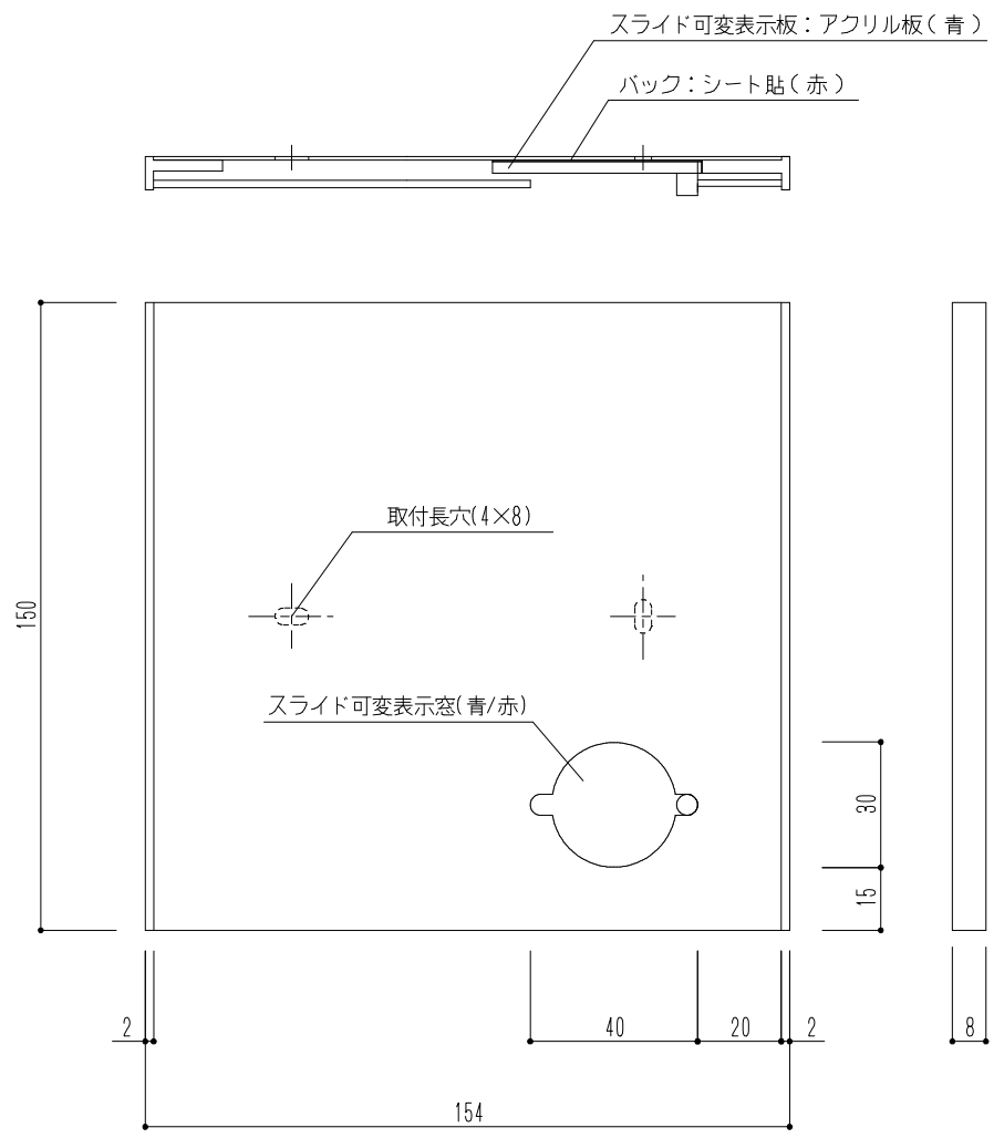
断面図
