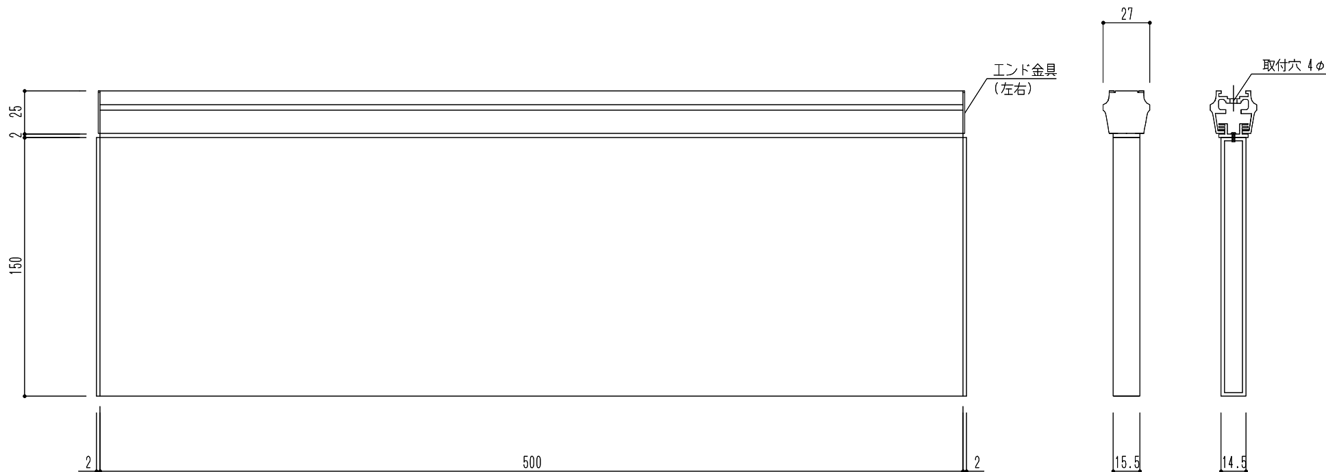
断面図
