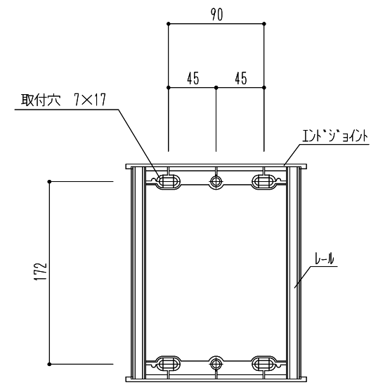
取付仕様
